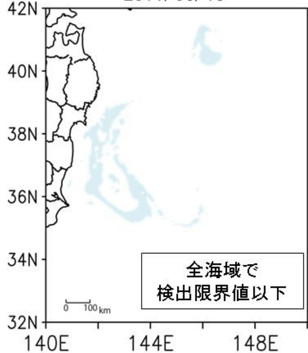
JCOPE2 予測値 (セシウム134) 2011/06/15
