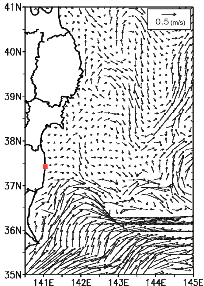
【図2】JCOPE2における流速分布（4月23日時点）
