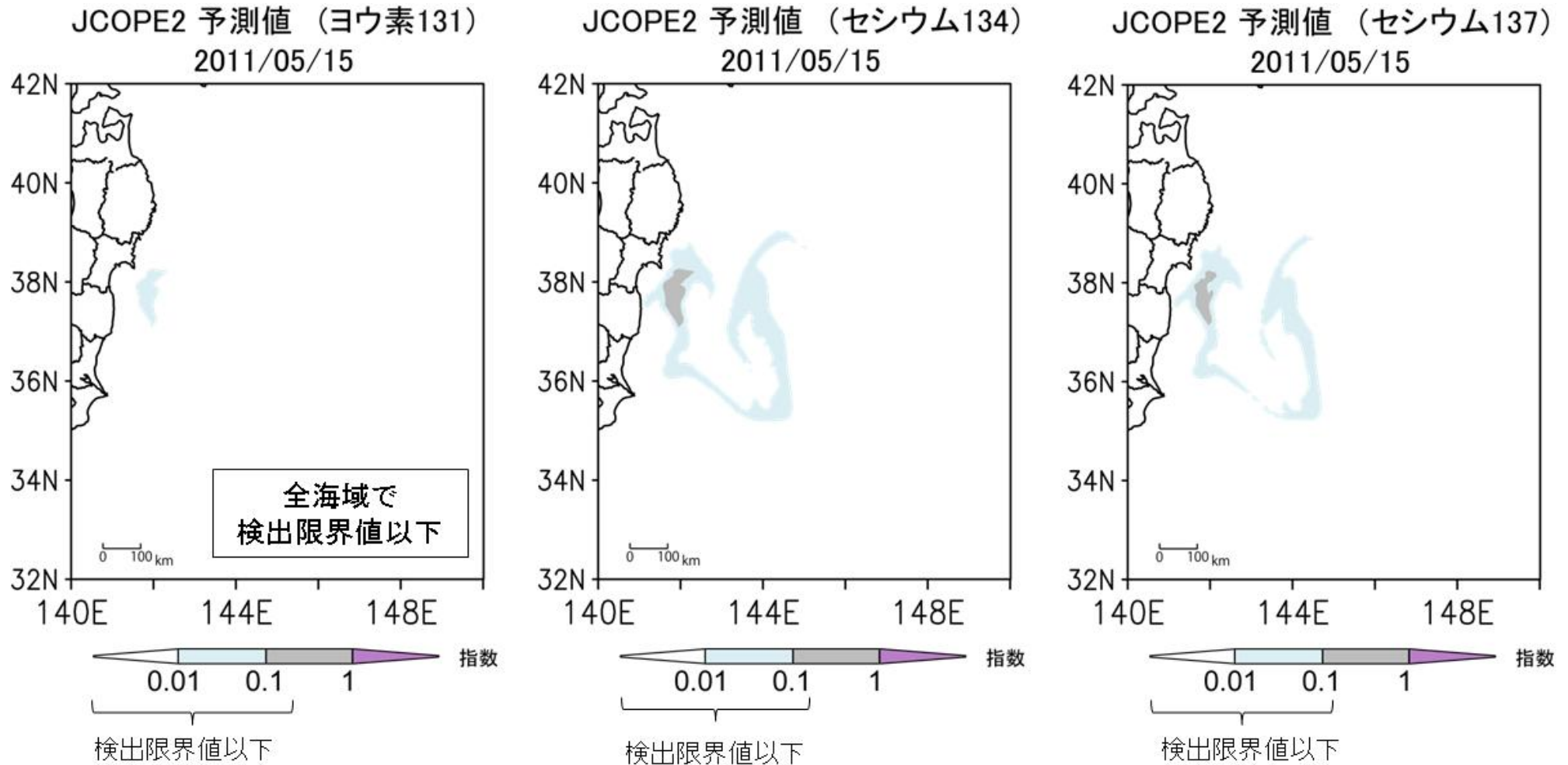
【図3-2】 JCOPE2による放射能濃度分布のシミュレーションー5月15日ー (4月23日までのデータに基づくシミュレーション)
