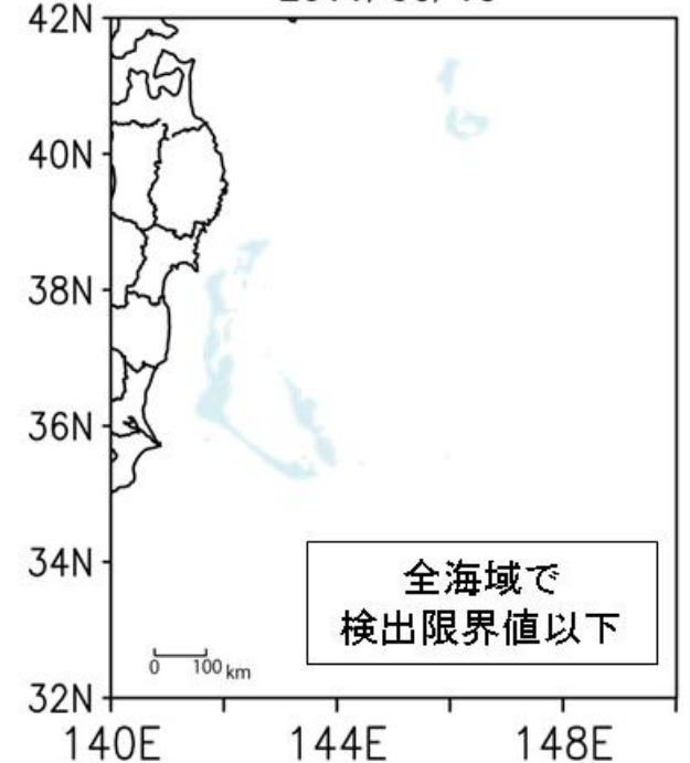
JCOPE2 予測値 (セシウム137) 2011/06/15
