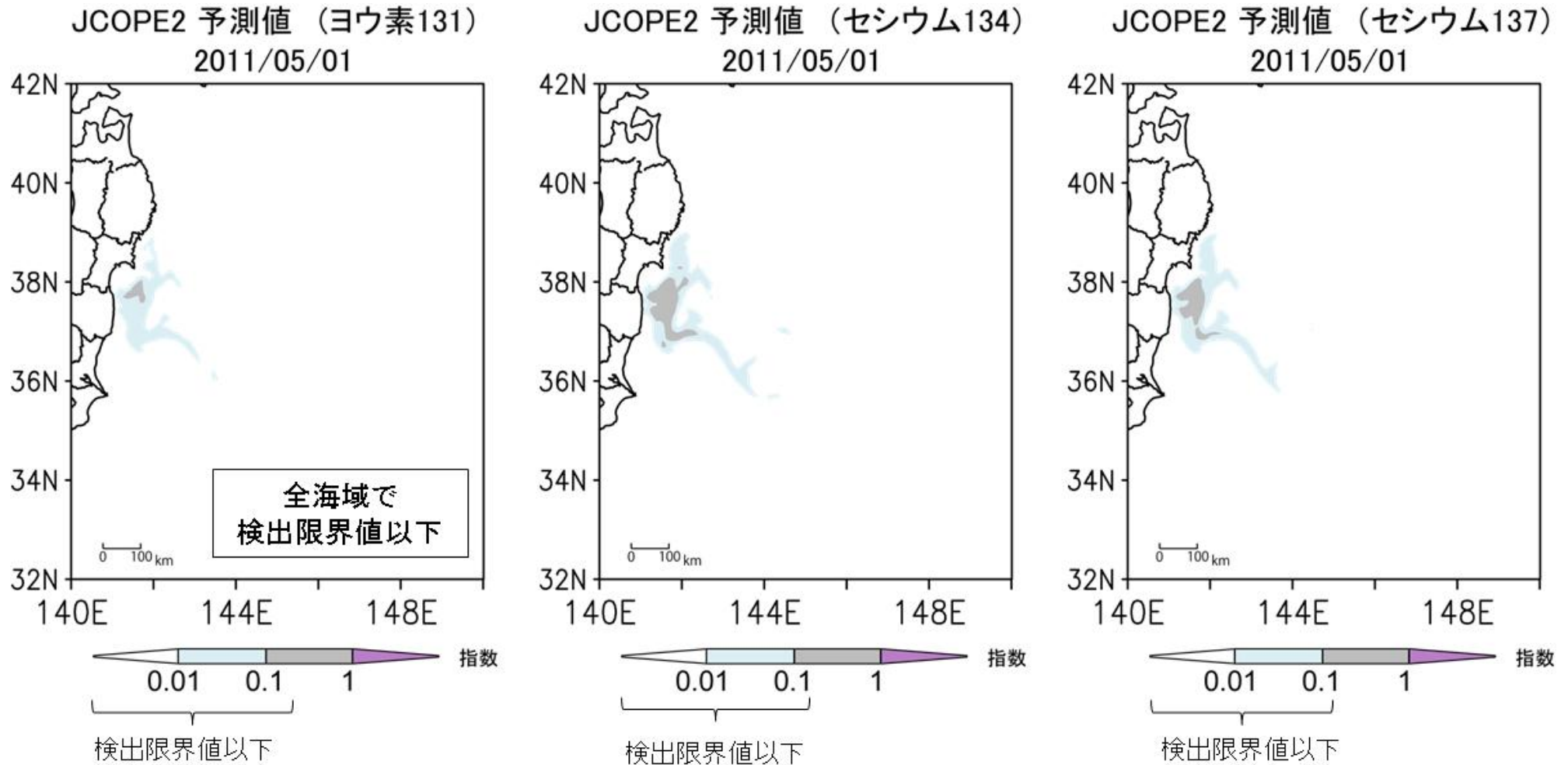
【図3-1】 JCOPE2による放射能濃度分布のシミュレーションー5月1日ー (4月23日までのデータに基づくシミュレーション)
