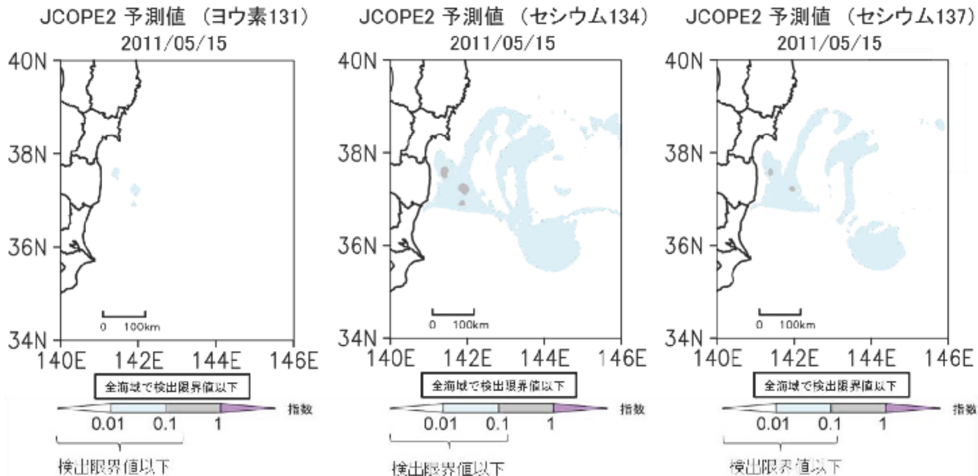
【図3-1】 JCOPE2による放射能濃度分布のシミュレーションー5月15日ー (5月3日までのデータに基づくシミュレーション)
