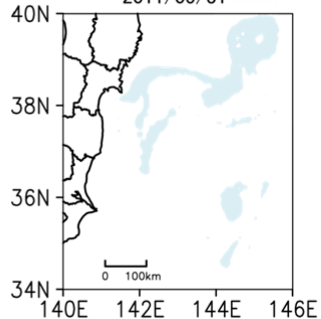
JCOPE2 予測値 (セシウム137) 2011/05/31
