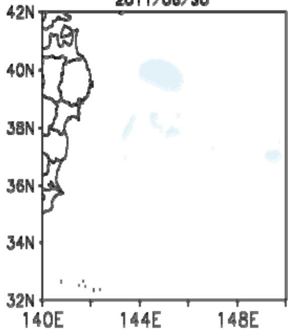
JCOPE2 予測値 (セシウム134) 2011/06/30
