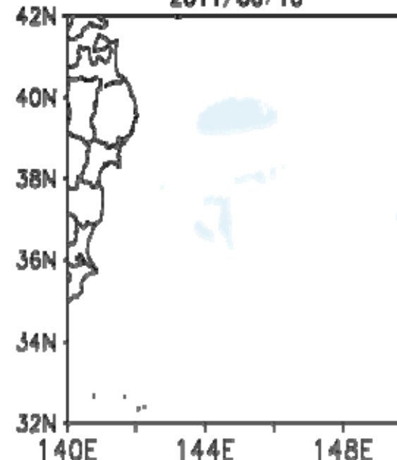
JCOPE2 予測値 (セシウム137) 2011/06/15
