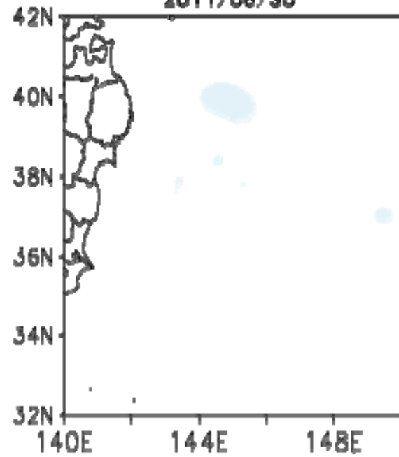
JCOPE2 予測値 (セシウム137) 2011/06/30
