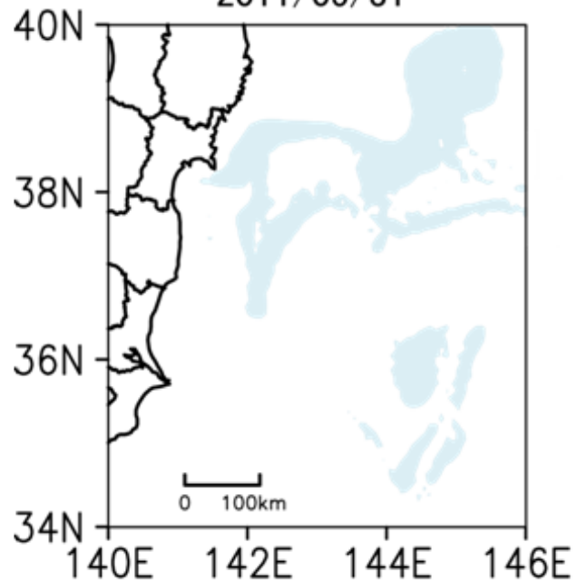
JCOPE2 予測値 (セシウム134) 2011/05/31
