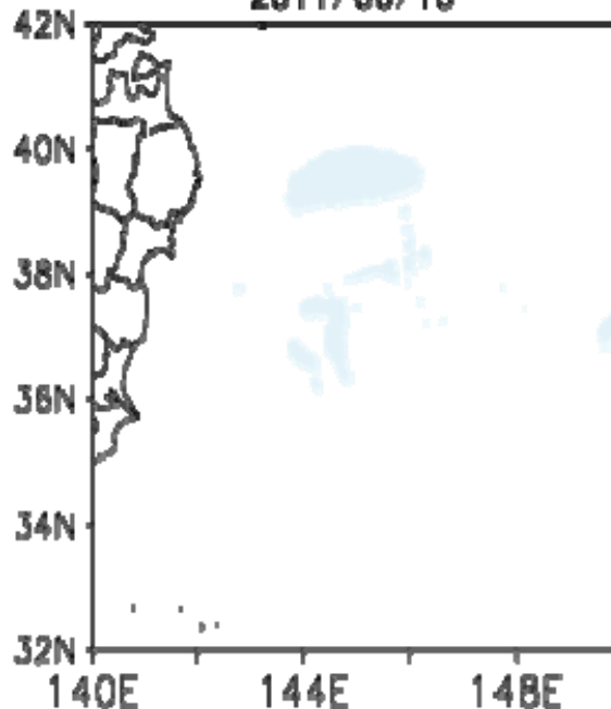
JCOPE2 予測値 (セシウム134) 2011/06/15
