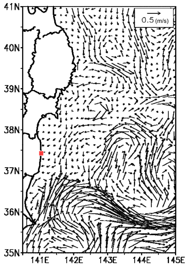
【図2】JCOPE2における流速分布(5月3日時点)
