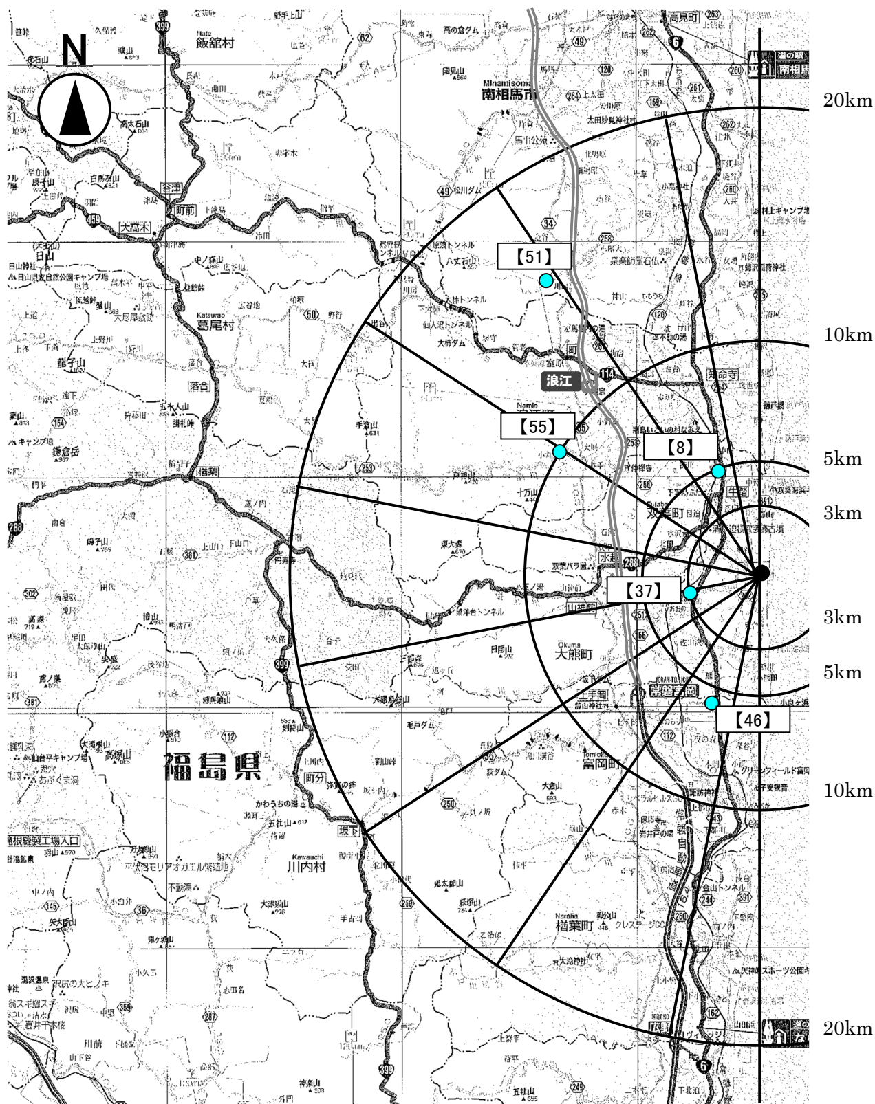
福島第一原子力発電所 20km 圏内の土壌試料採取ポイント（試料採取日：令和 6 年 9 月 3 日）
