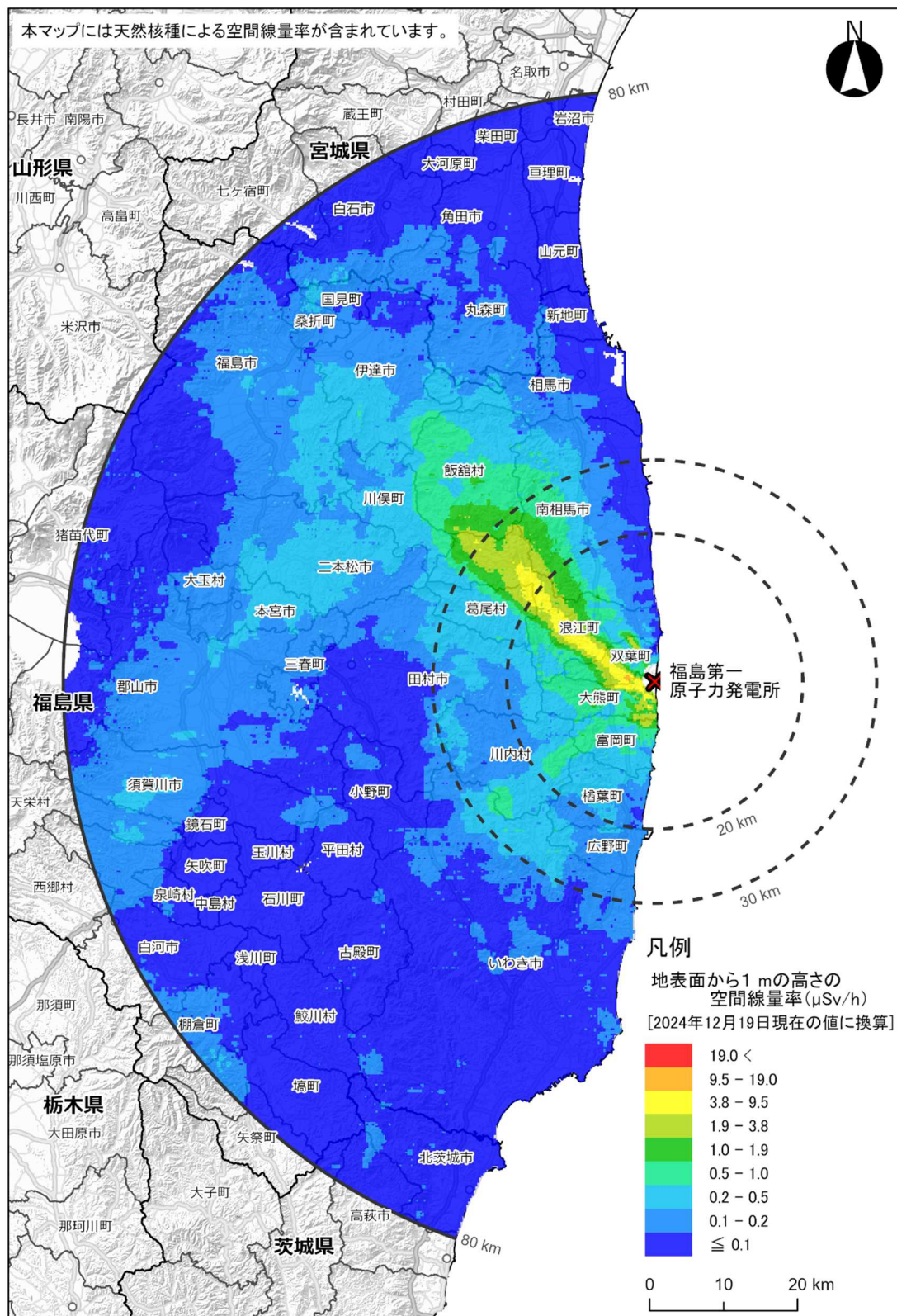
80 km 圏内における空間線量率の分布マップ (2024年12月19日時点(事故から約165か月後))
